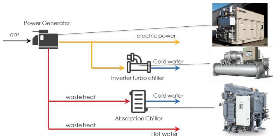
Fig. 5.3-9. Co generation system
